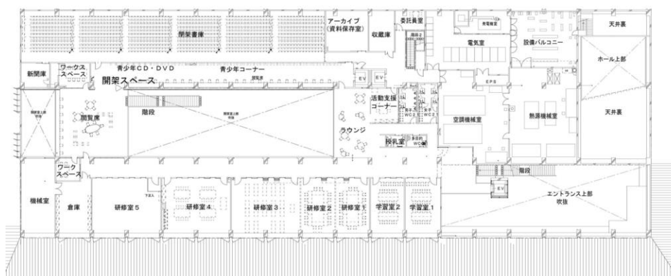
2階平面
